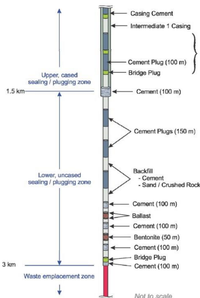
Figure 4 : Structure complète du stockage ( Brady.PV 2017 Gibb, F., 2024)
